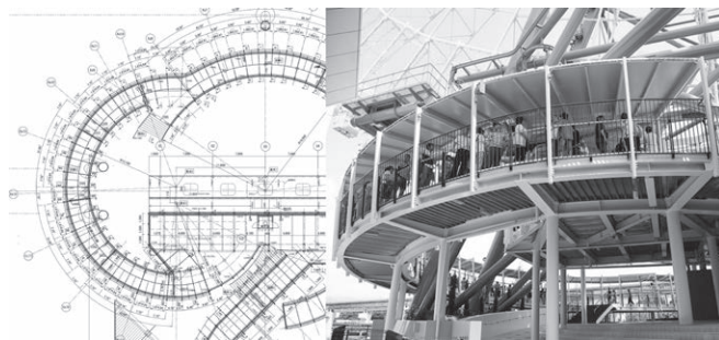
※大阪ホイール コリドール実施設計
